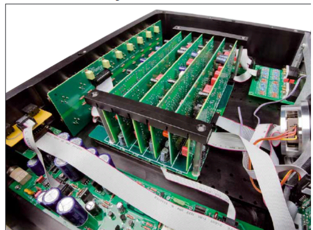
Die Technik der Momentum-Vorstufe ist zum größten Teil auf sechs Steckkarten verteilt
